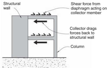
End elevation
